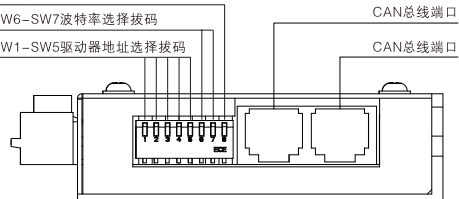
SW8 120终端电阻选择拨码
