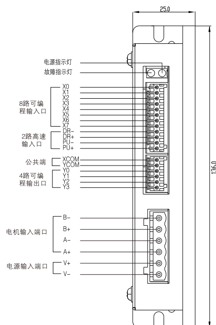
驱动器接线示意图
