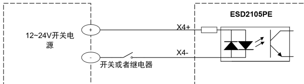
差分信号 X4 接入到开关或继电器
