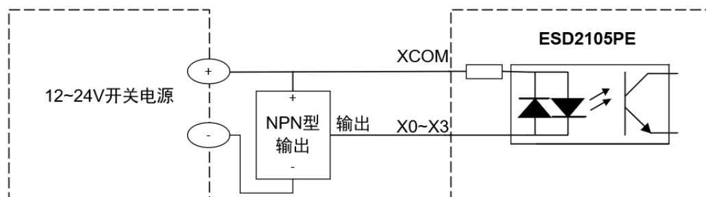
将 X0-X3 接入到 NPN 输出
