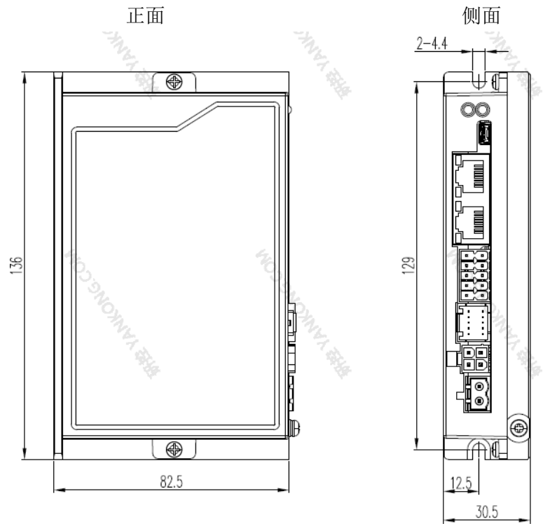
安装尺寸图（单位：mm）
