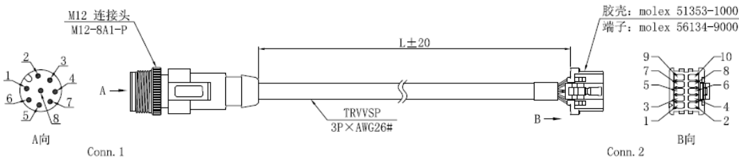
编码器线引脚定义
