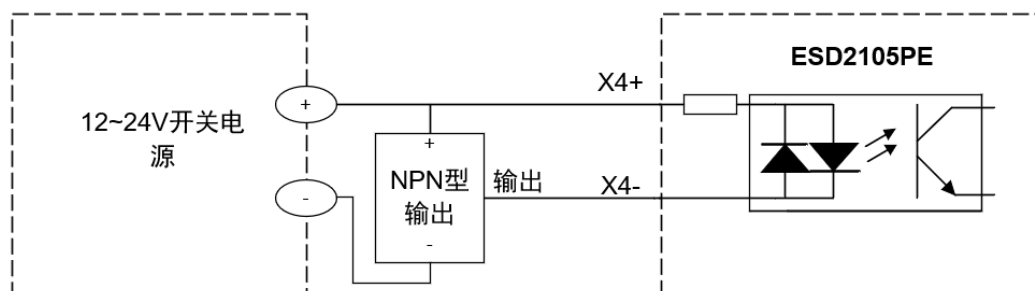
差分信号 X4 接入到 NPN 输出
