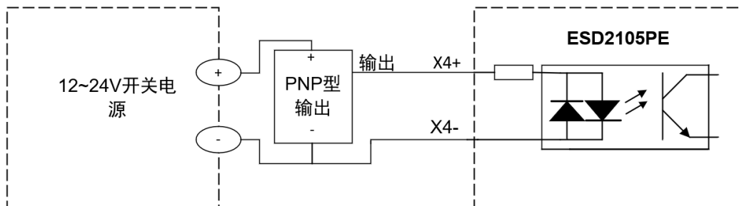
差分信号 X4 接入到 PNP 输出
