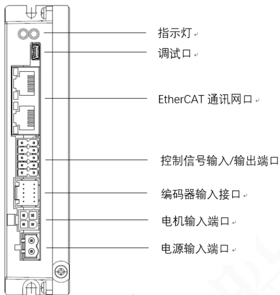
驱动器接线示意图
