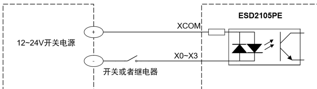
将 X0-X3 接入到开关或继电器
