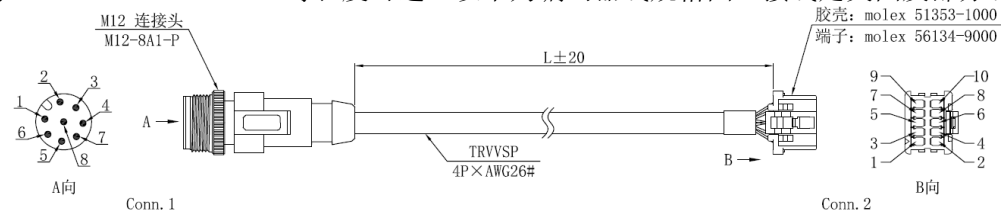
编码器线引脚定义
