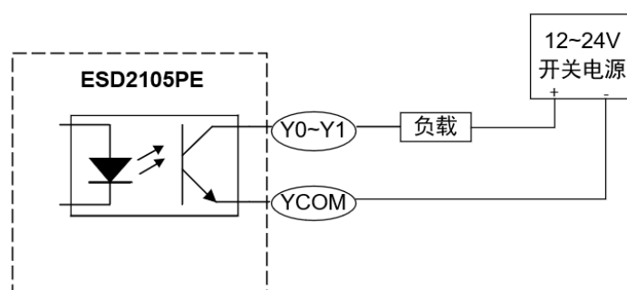
将 Y0~Y1 接成 sinking 型输出
