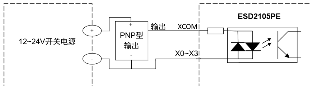
将 X0-X3 接入到 PNP 输出
