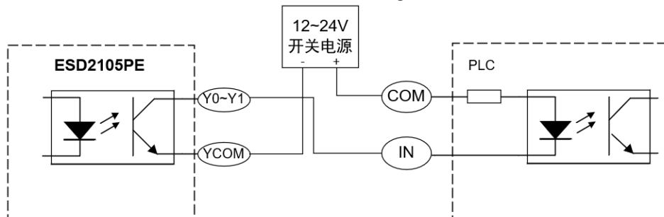
将 Y0~Y1 接成 sinking 型输出，连接到 PLC
