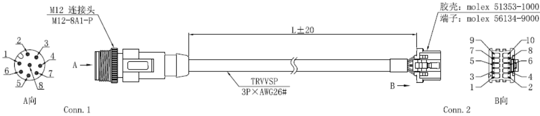
编码器线引脚定义
