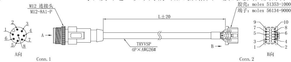
编码器线引脚定义
