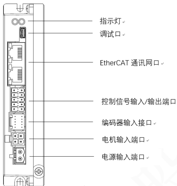
驱动器接线示意图
