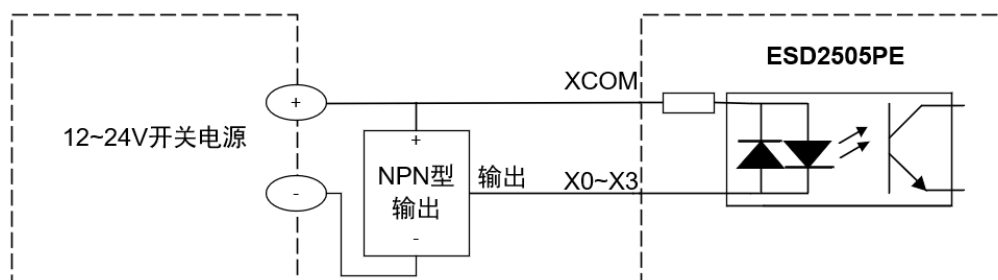
将 X0-X3 接入到 NPN 输出
