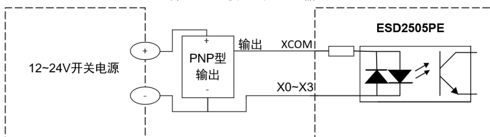
将 X0-X3 接入到 PNP 输出
