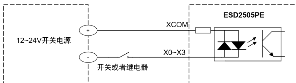
将 X0-X3 接入到开关或继电器
